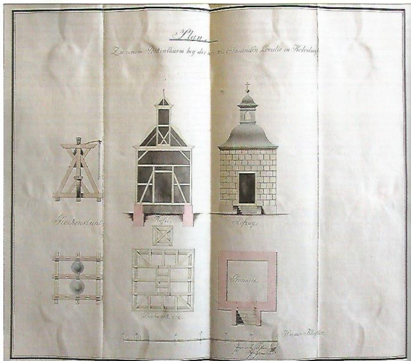
Obr. 2: Návrh zvonice u nové budovy lokálního kaplana v Kolodějích, inženýr Ignatz Schmid [březen 1805] (SLHA, sign. A1-1/18, nefol.).
